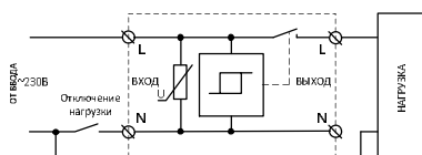
Рис. 1в
