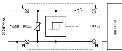
Рис. 1а
