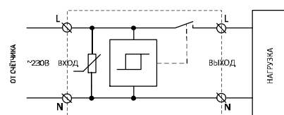
Рис. 1б
